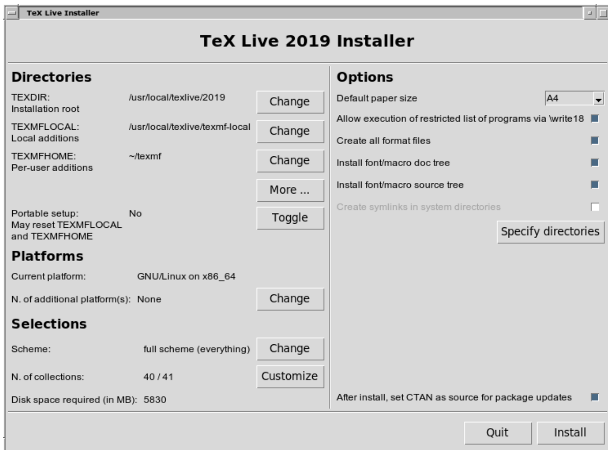
图 4: 高级 GUI 安装界面 (GNU/Linux)
