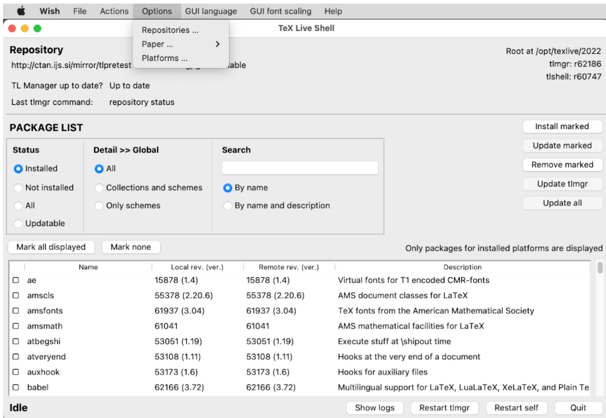
Abbildung 6.1: tlmgr GUI, mit dem Auswahlmönü (Mac OS X)
